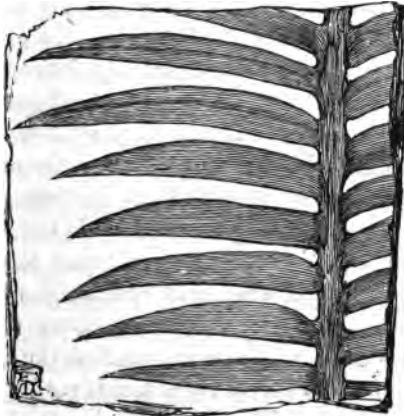
ZAMIA FENDLERI. (Portland Oolite.)
